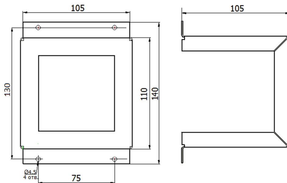
Рисунок 2 - Габаритные размеры защитного кожуха
